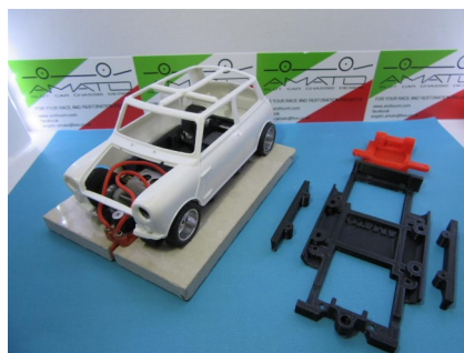
Mini 1:24th Front Wheel Drive
